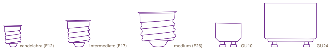
candelabra (E12)
